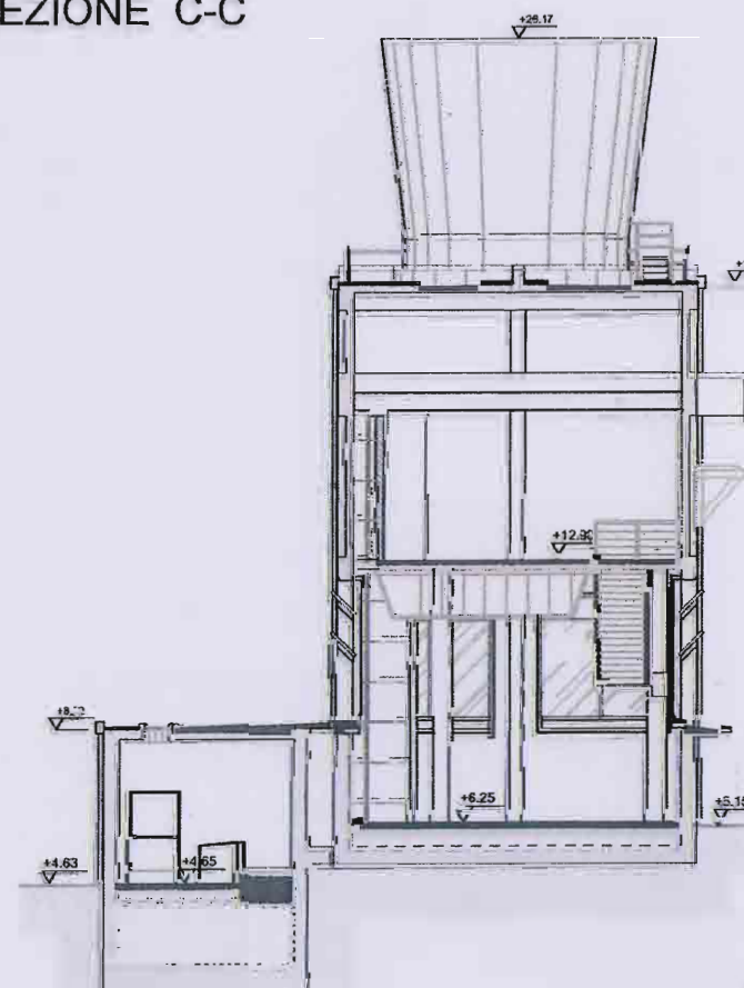
SEZIONE C-C
